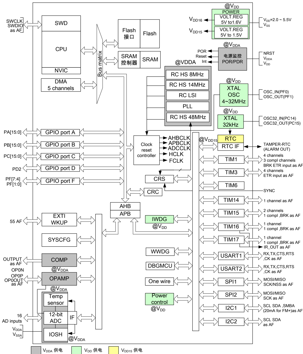
图 2-1 系统框图
