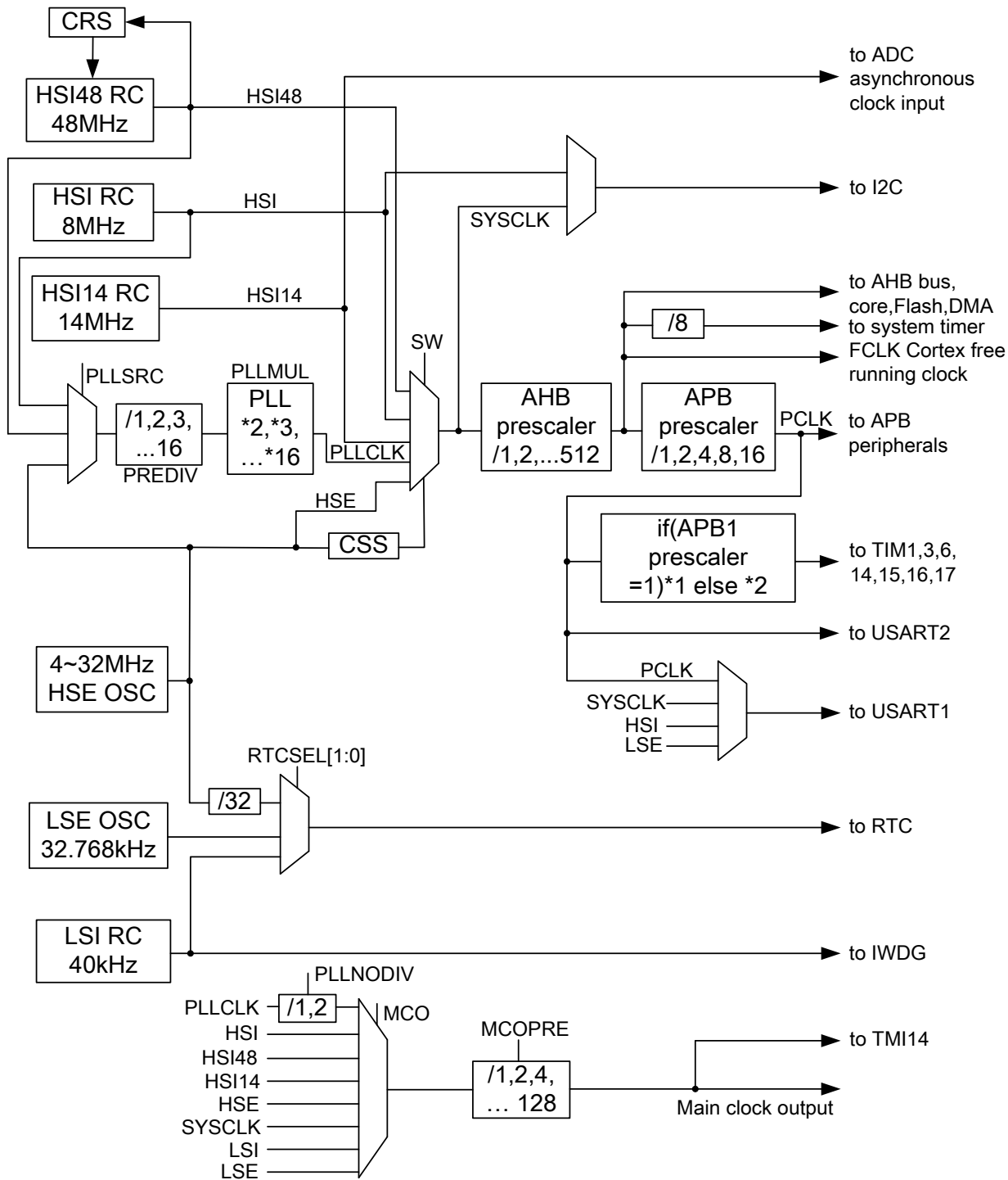
图 3-1 时钟框图
