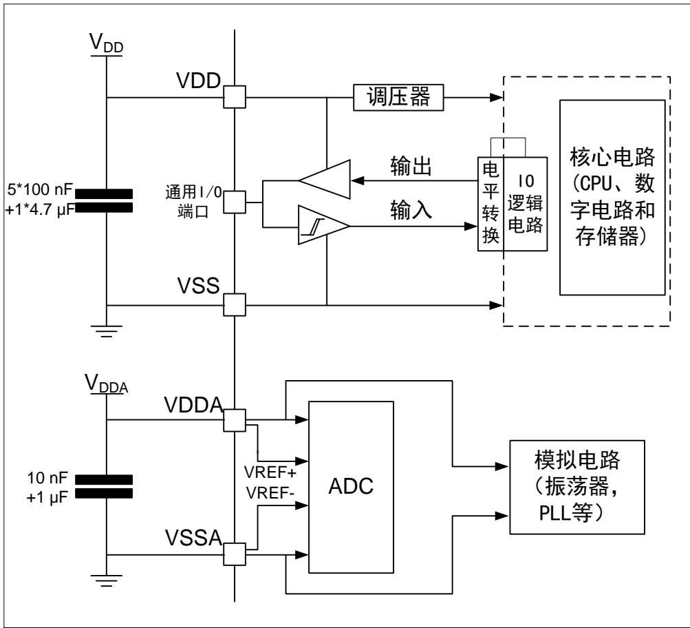
图 6-3 供电方案图
